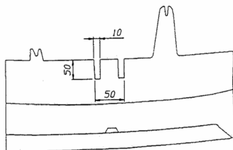
Obr. 3 Výřez dolní části nárazníku
